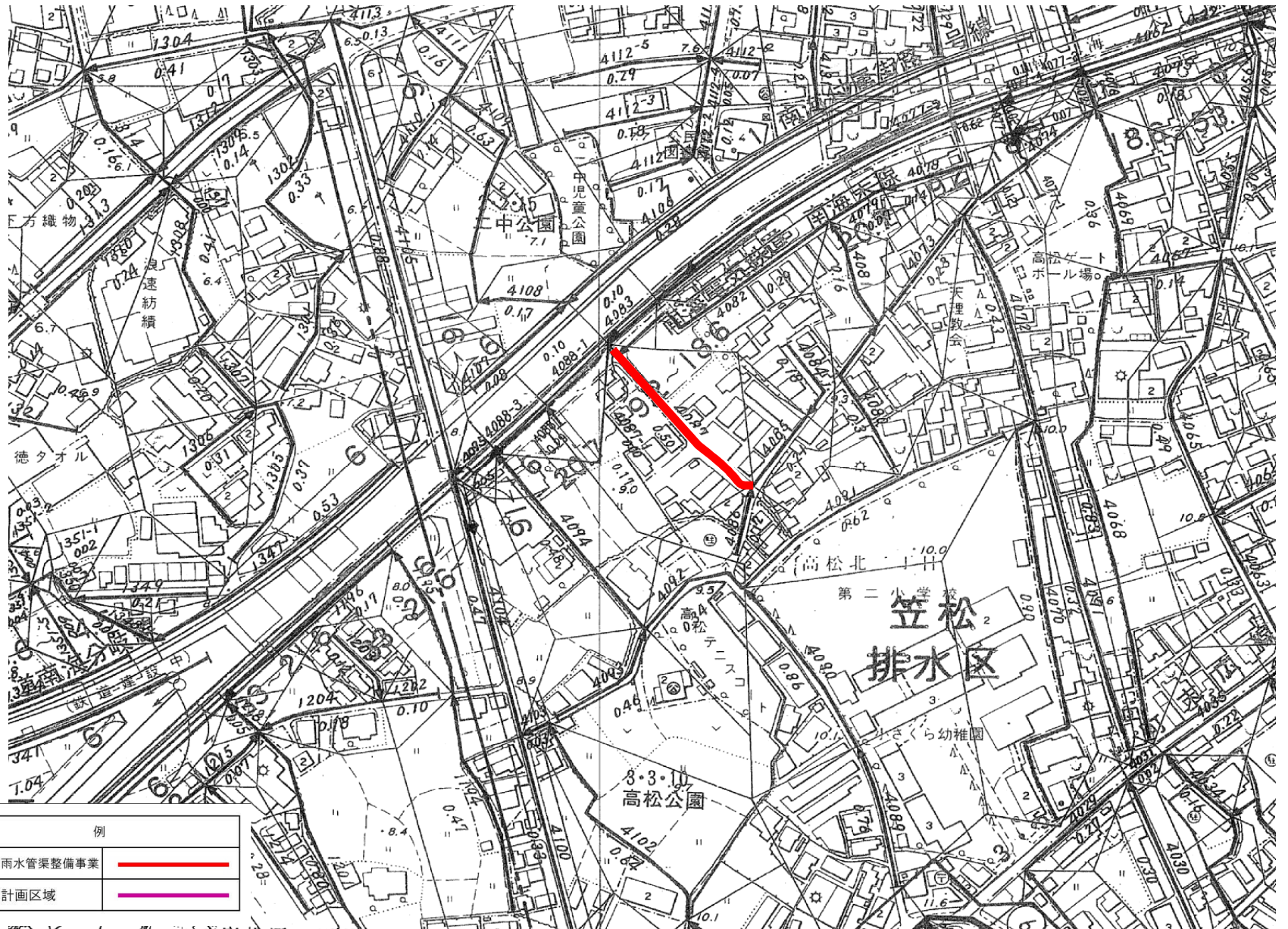
(参考図面) 雨水詳細図2
