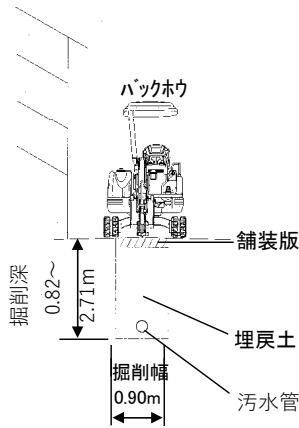
開 削 工 標 準 図
