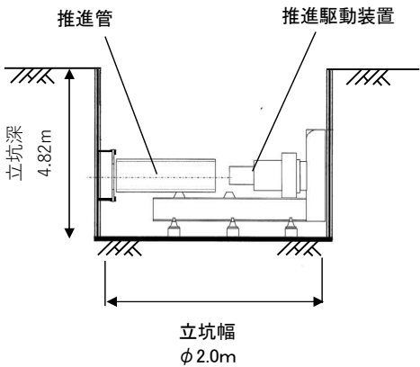
推 進 工 標 準 図
