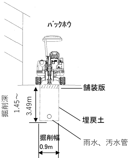
開削工標準図
