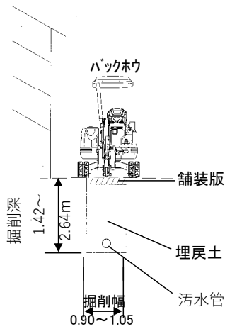
開削工標準図
