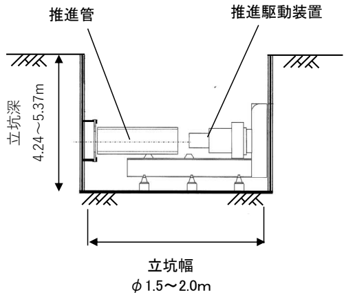
推進工標準図
