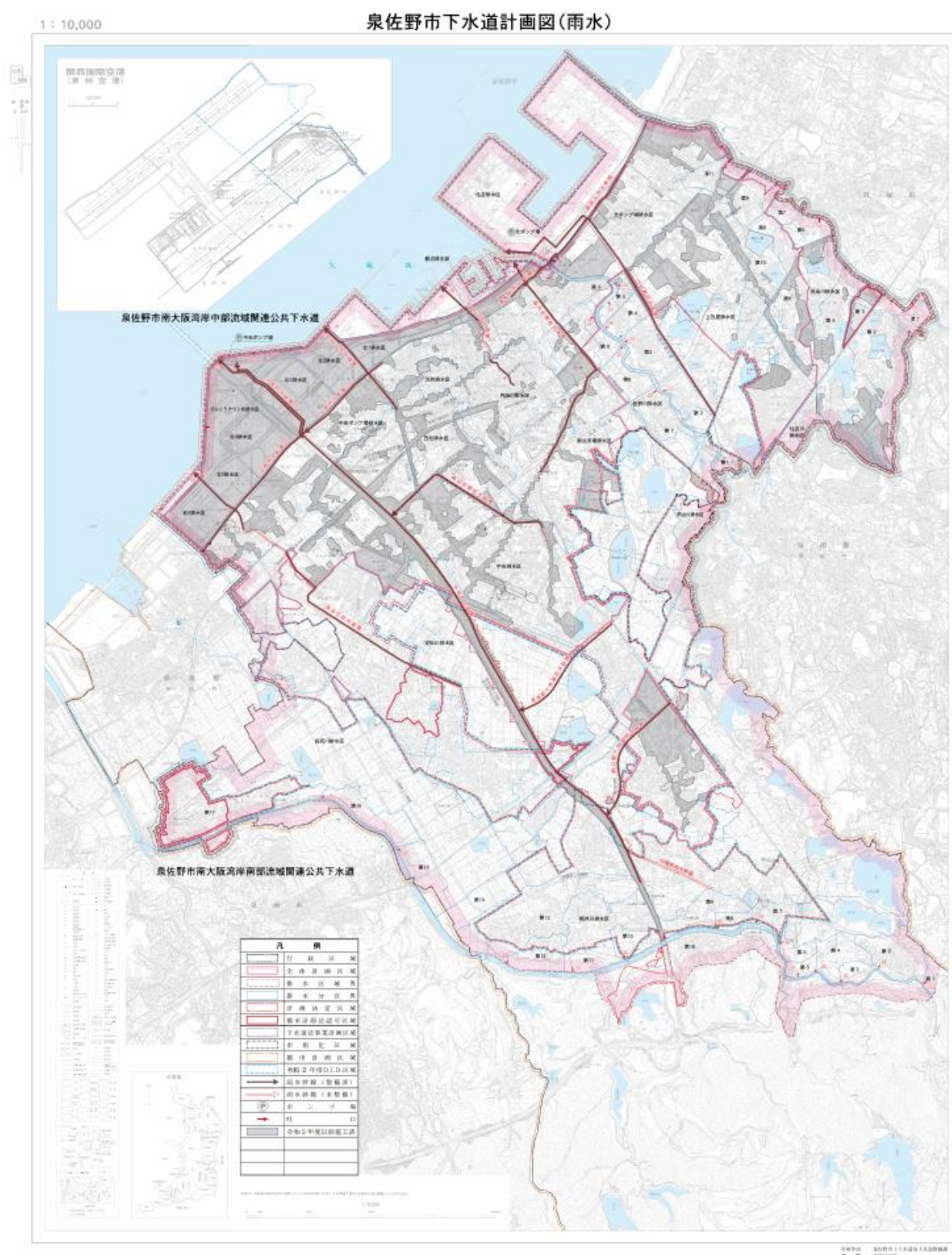
図表 2-1-4 下水道計画一般図（雨水）
