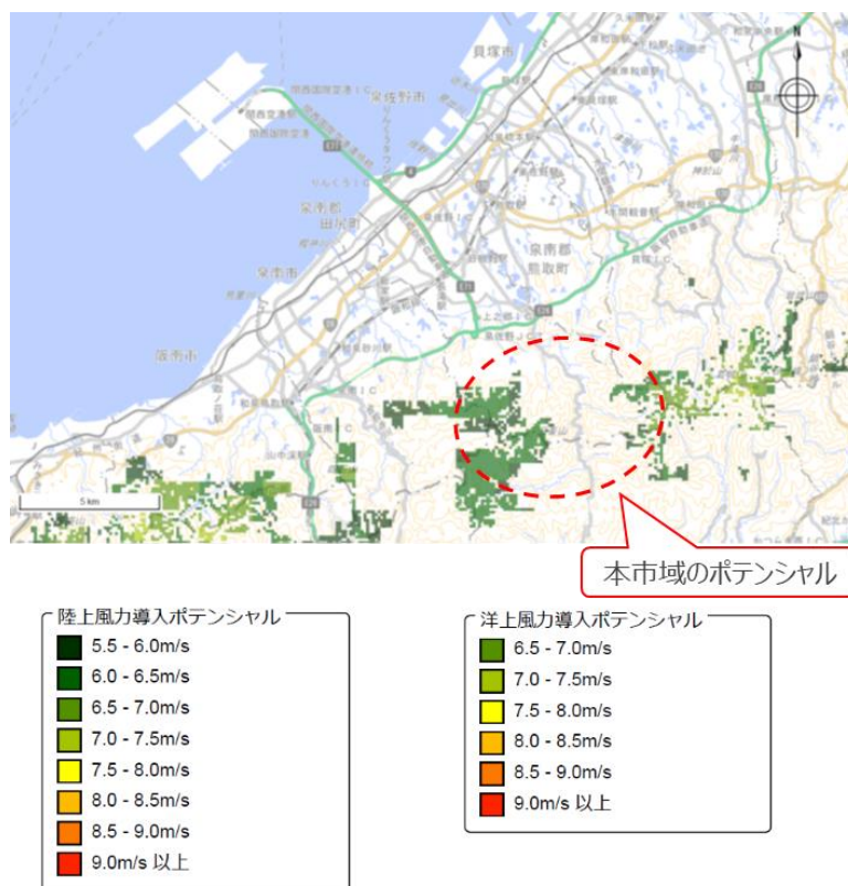
風力発電のポテンシャルマップ (出典) 環境省「REPOS」
