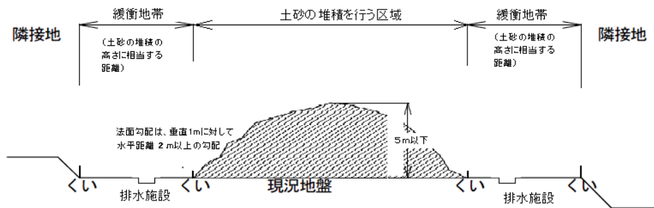
解図 15-2-1 一般的な一時堆積
