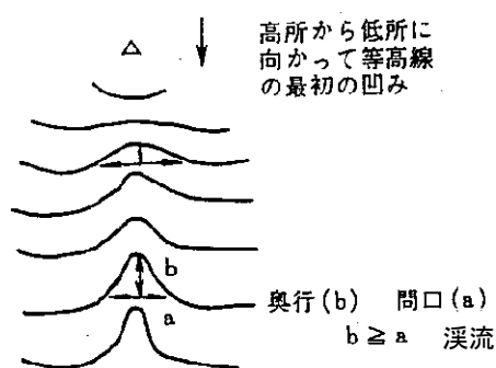
解図 7-3-1 溪流の定義 2)
