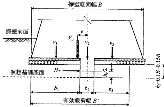
参図 7-5-2 突起を設けた場合の滑動に対する安定 8)
