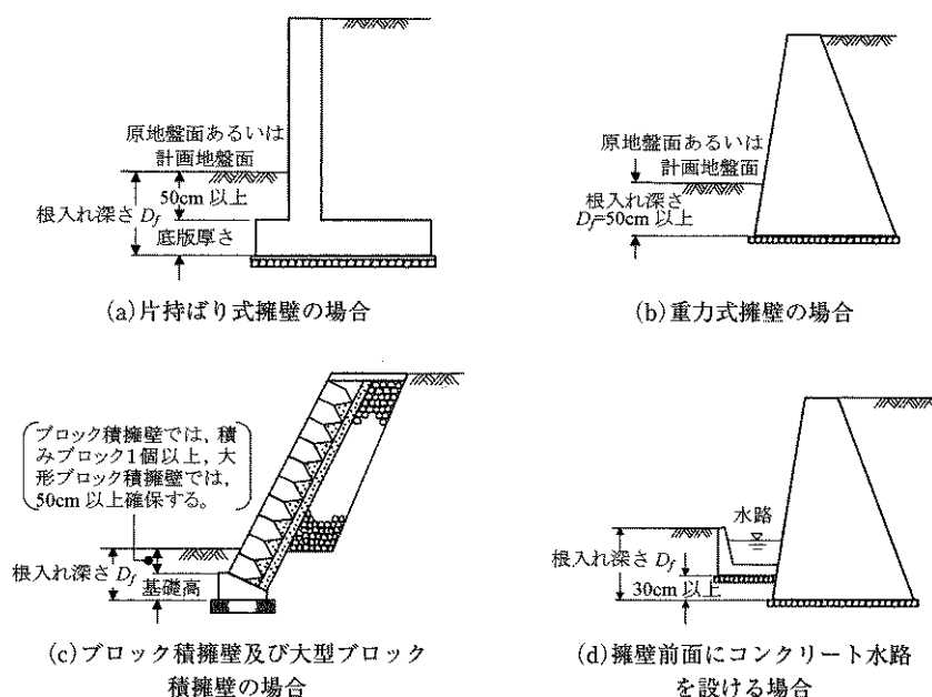
解図 7-5-12 擁壁の直接基礎の根入れ深さ 8)
