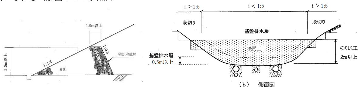
解図 7-1-2 法尻工の基本形状 12) を一部修正
