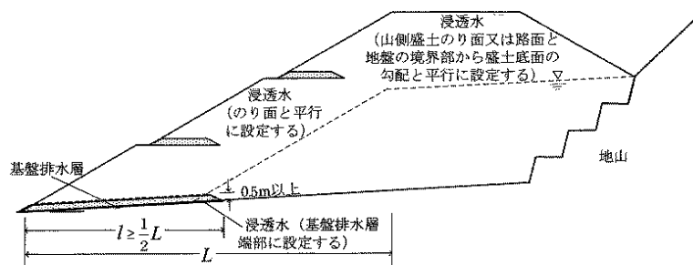
解図 4-2-4 地山から浸透流の簡易設定法 6)
