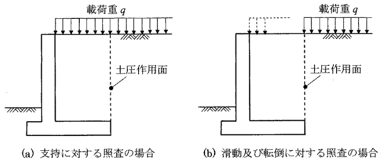
解図 7-5-8 嵩上げ盛土形状が変化する場合の \beta' の設計方法 8)
