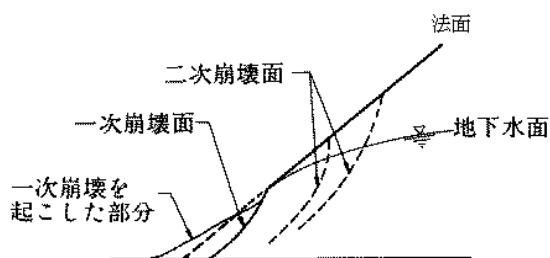
解図 7-1-1 盛土法面の一次と二次崩壊の例 6)
