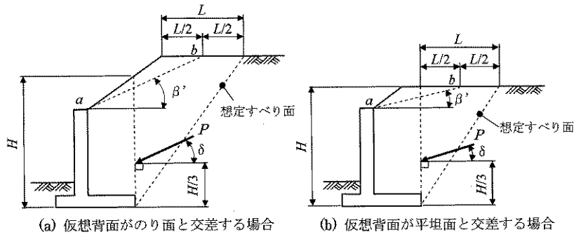
解図 7-5-7 嵩上げ盛土形状が変化する場合の \beta' の設計方法 8)
