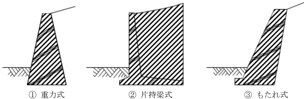
解図 7-5-1 自重の考え方 3)
