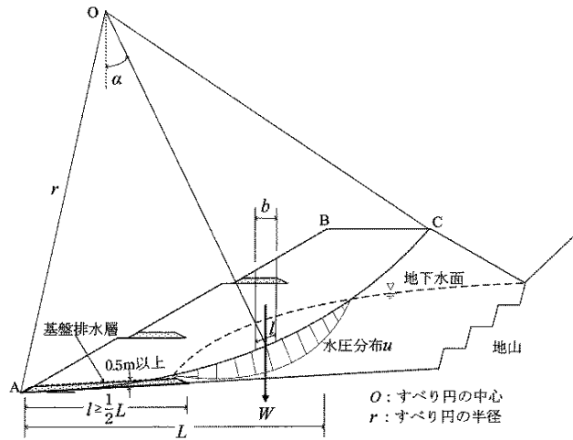
解図 4-2-3 浸透流のある盛土の安定解析 6)
