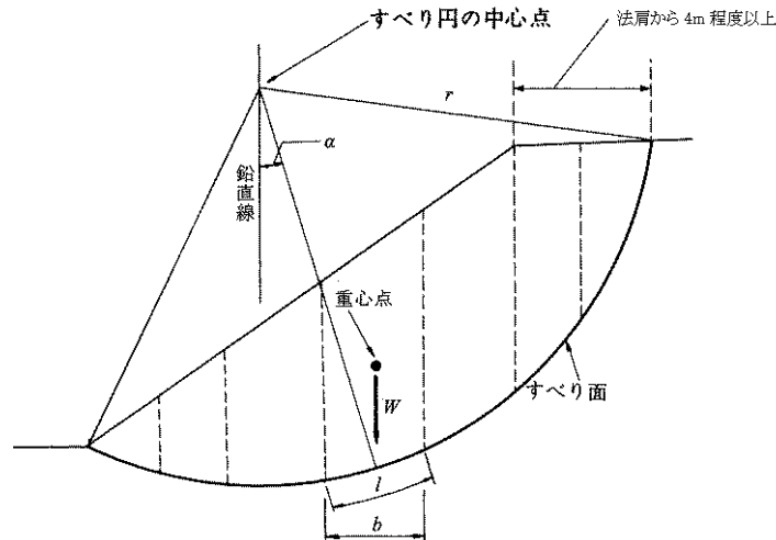
解図 4-2-5 レベル 2 地震動に対するすべり面の設定 6) を一部修正
