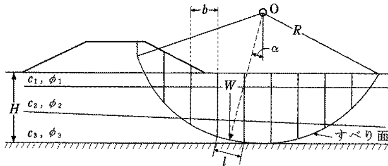
解図 4-2-6 分割法による安定計算 7) を一部修正
