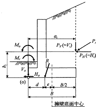
解図 7-5-10 合力作用位置の求め方 8)
