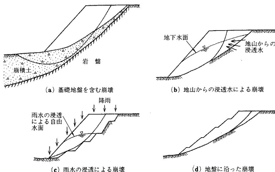
解図 3-1-1 傾斜地盤における盛土の崩壊パターン 12)
