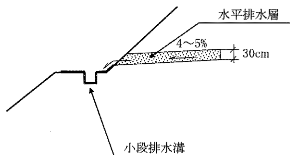
解図 8-2 水平排水層端末部 12)
