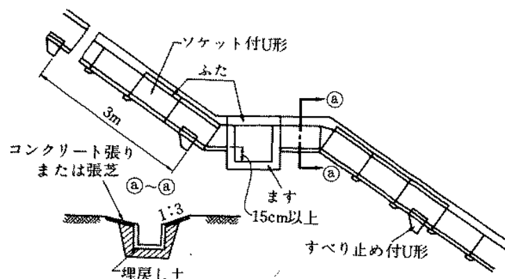
解図 9-2 縦断排水溝 6)
