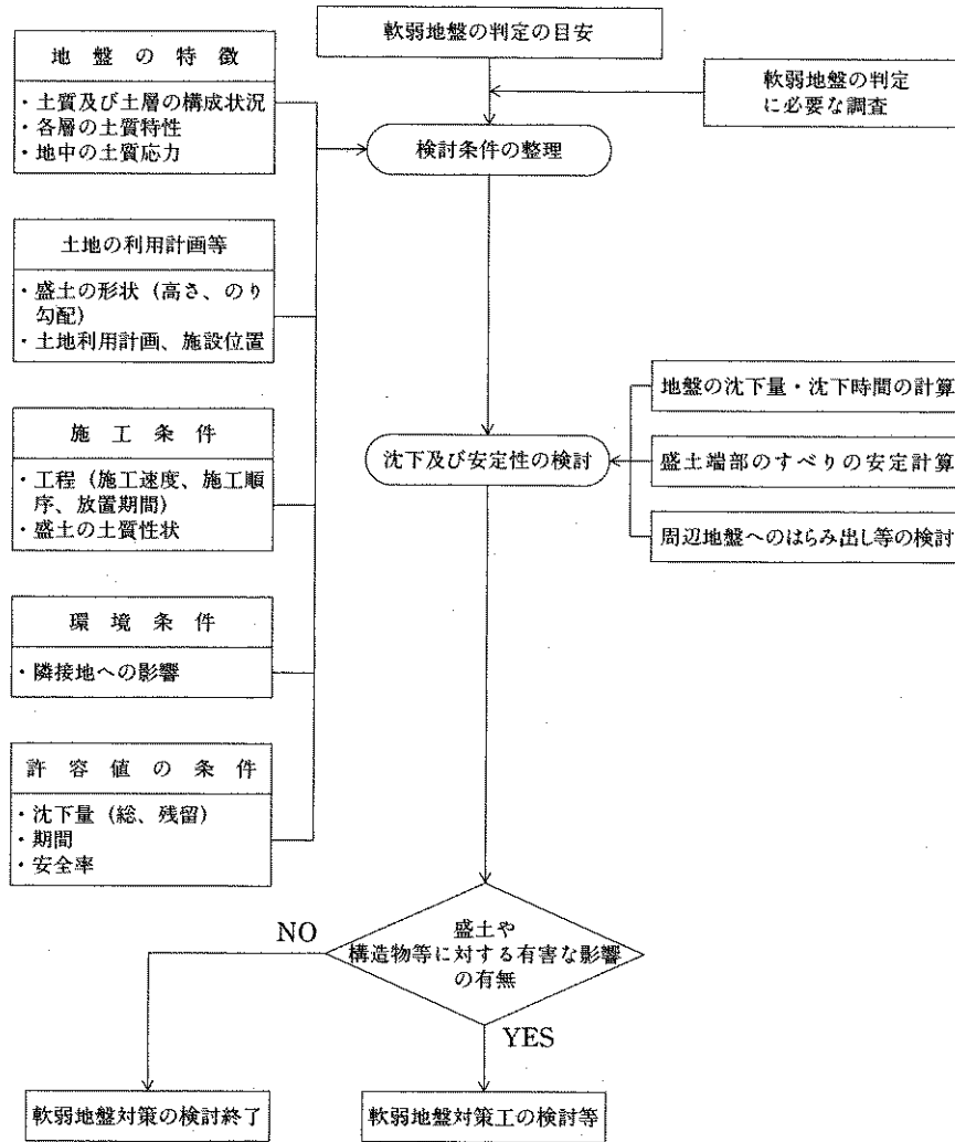
解図 2-3-1 软弱地盤対策の検討の流れ 11)
