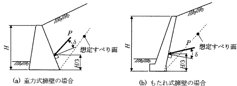
解図 7-5-5 重力式擁壁等の土圧作用面 8)
