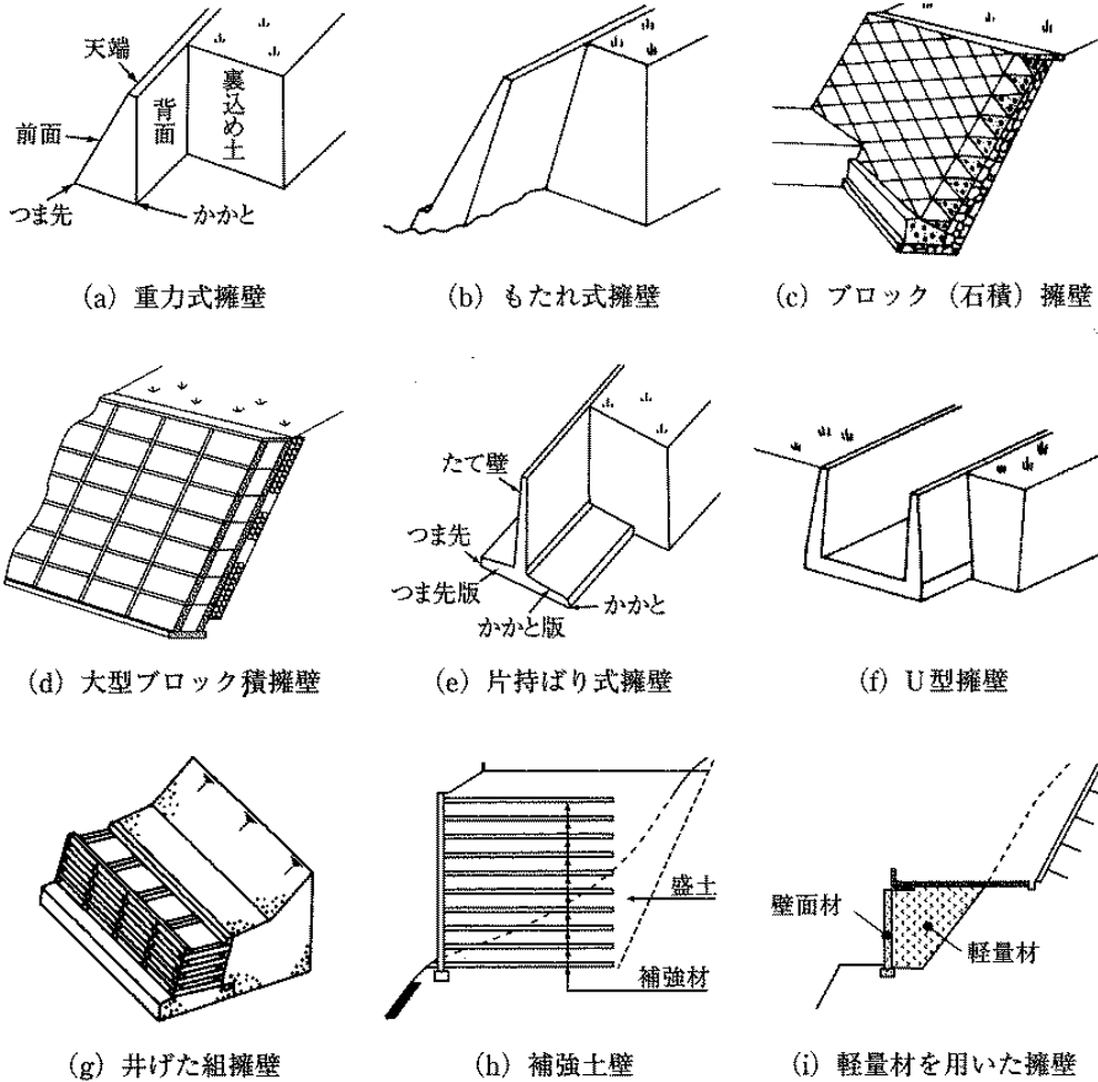
解図 7-2-1 擁壁の形式 8)
