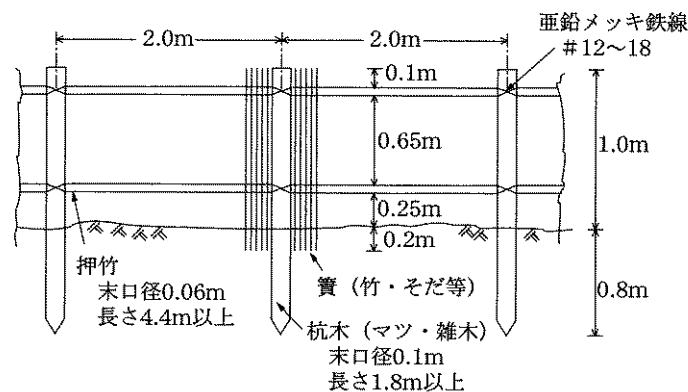
解図 14-1 標準施工図（静砂垣） 19)
