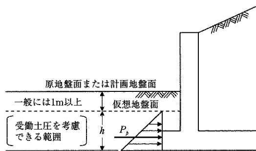
参図 7-5-1 擁壁の前面地盤による受働土圧 8)
