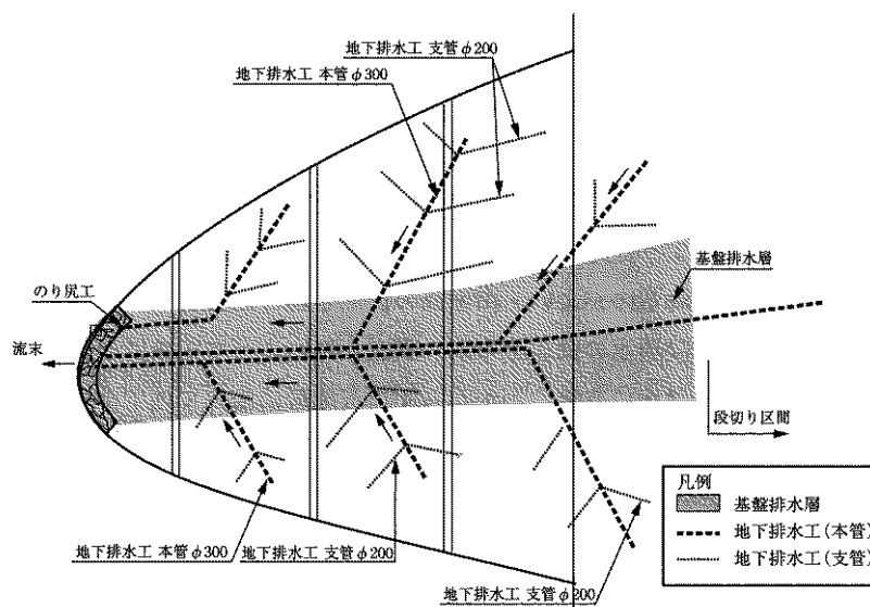
解図 6-1-1 沢埋め盛土における地下排水工及び基礎排水層の設置例 6)
