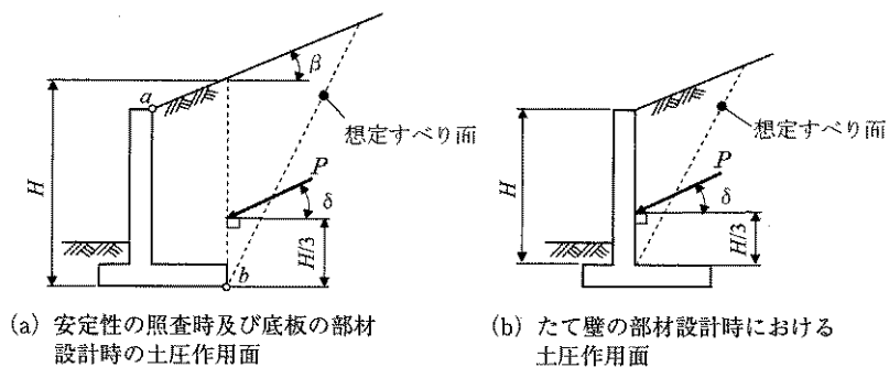
解図 7-5-6 片持ばり式擁壁等の土圧作用面 8)
