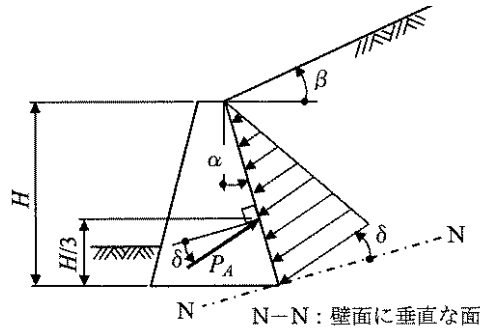
解図 7-5-3 主働土圧の角度の取り方 8)
