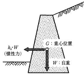
解図 7-5-10 擁壁の慣性力の考え方 8)
