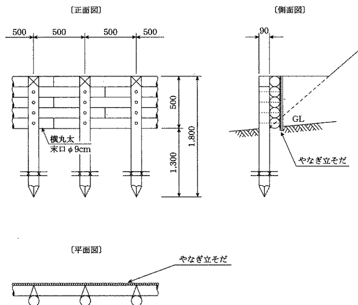
解図 14-2 標準施工図（柵工） 19)
