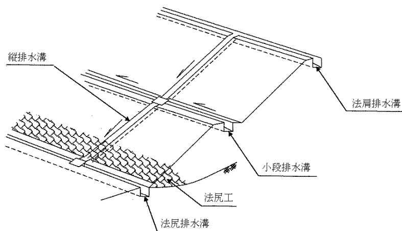
解図 9-1 法面排水施設の概念図 12)
