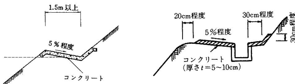
解図 8-1 小段排水溝の例 9)
