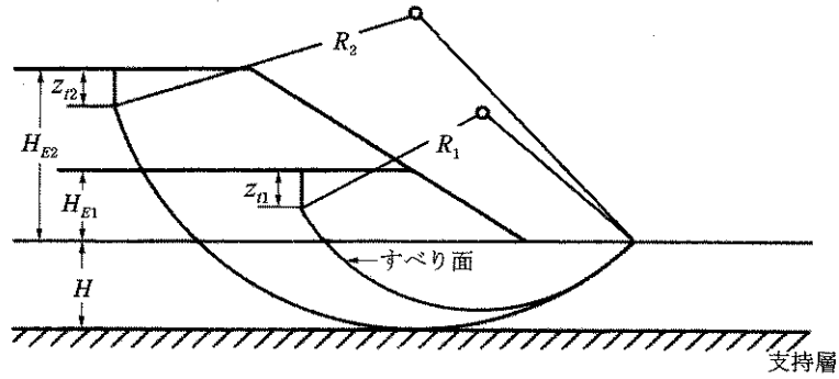
解図 4-2-7 高い盛土の安定計算 7)を一部修正
