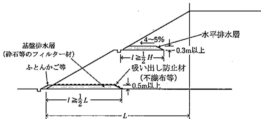
解図 6-1-3 水平排水層及び基盤排水層の例 6)
