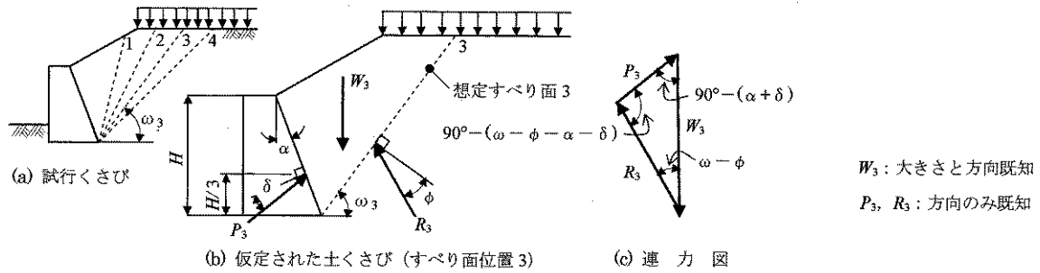
解図 7-5-2 試行くさび法による土圧図解法 8)
