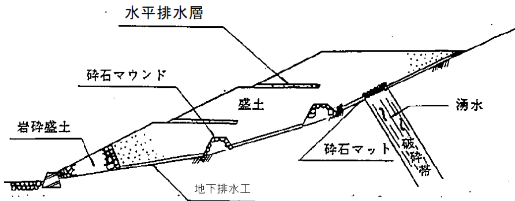
解図 6-2-2 排水対策の一例 2) を一部修正
