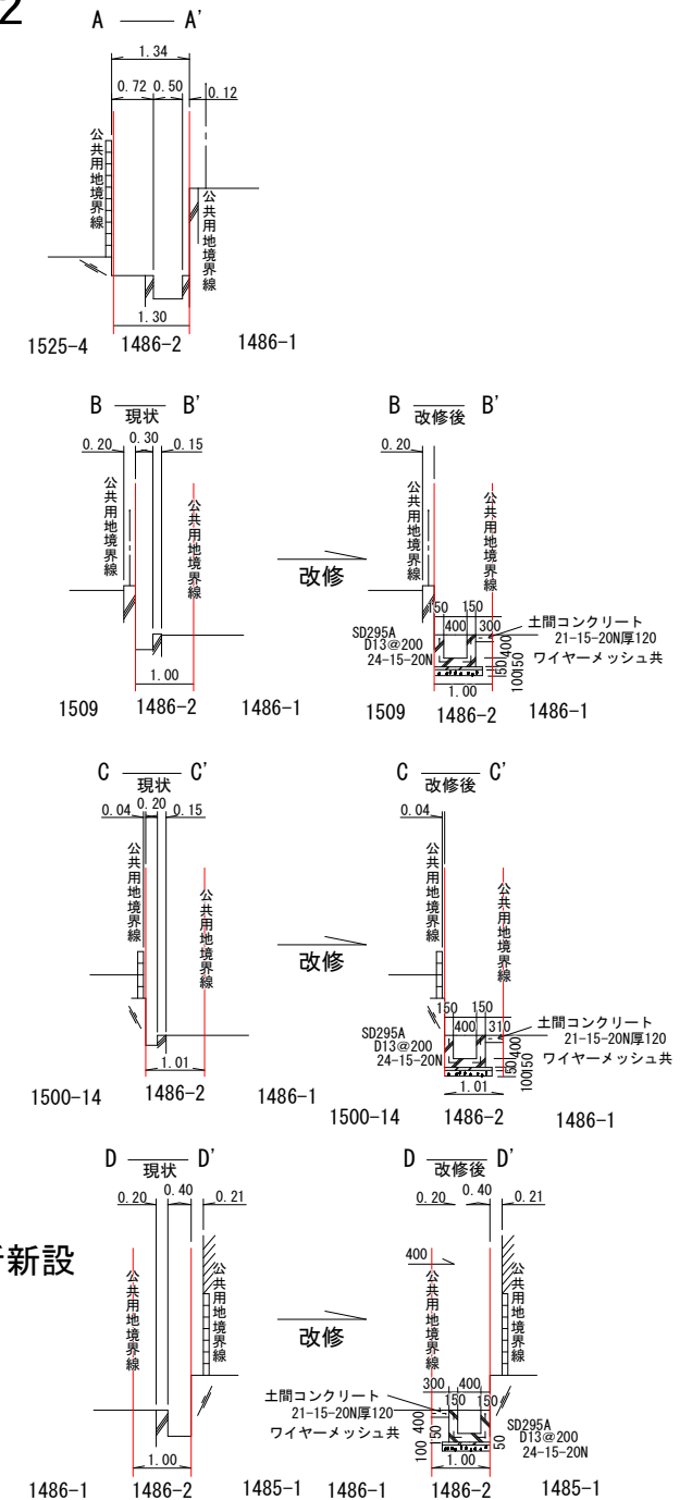
横断面図
