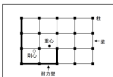
RC造ラーメン構造の駐車場 ピロティ型マンション
