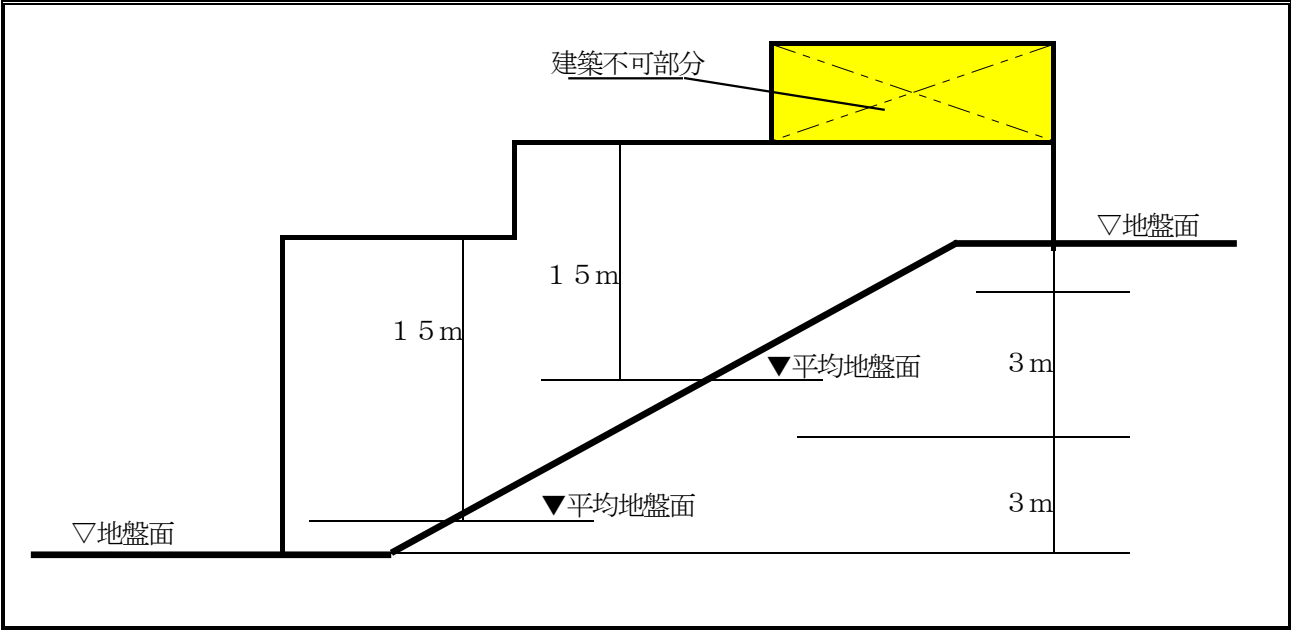
図ー 1（土地の高低差がある場合の建築物の高さの算定）
