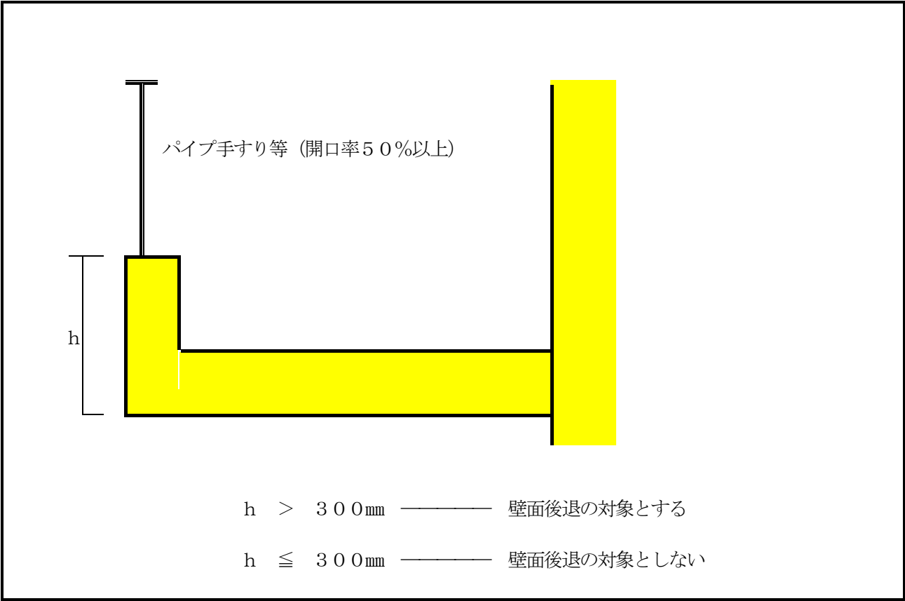
図ー 2（外壁後退の壁面とみなさないことができるバルコニー（ベランダの類を含む）の形態）
