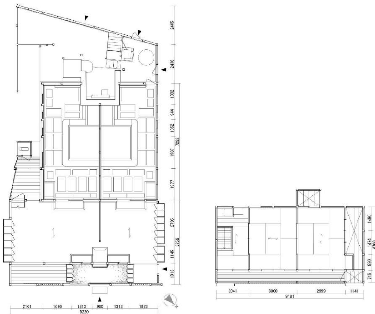
図0-4 大將軍湯平面図
