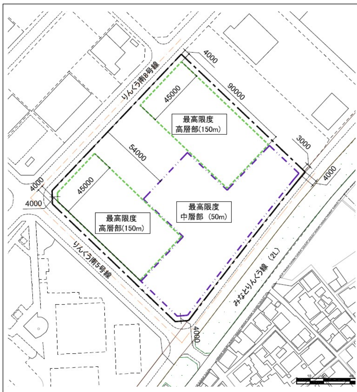
計画図
